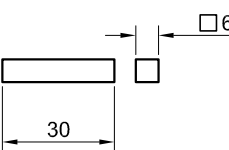
KEY [5]
